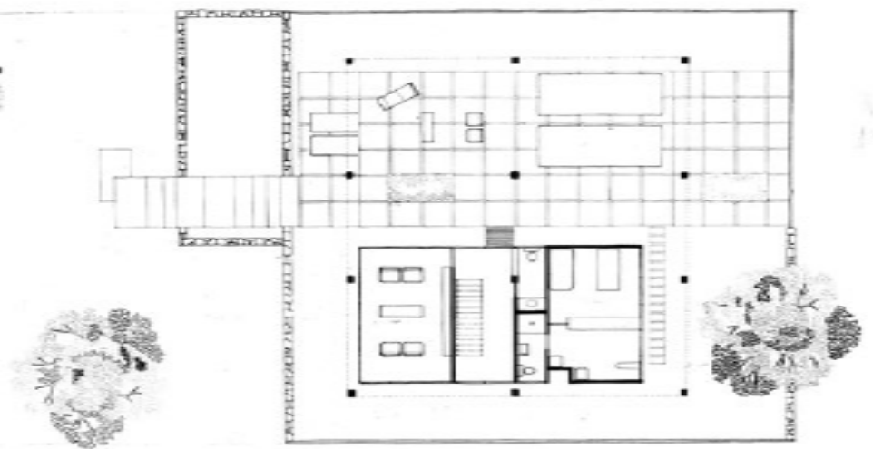
Club de Golf Hacienda, planta baja y planta alta. Estado de México.
